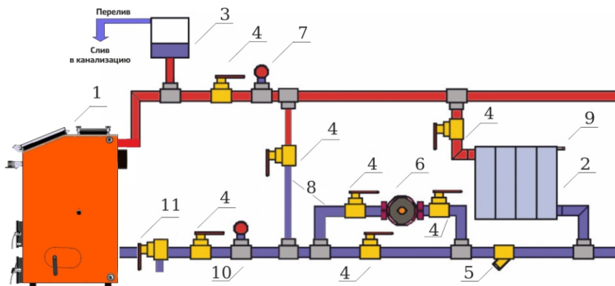
Рис.№8 Подключения котла к 2-х трубной открытой системе с принудительной циркуляцией теплоносителя:
