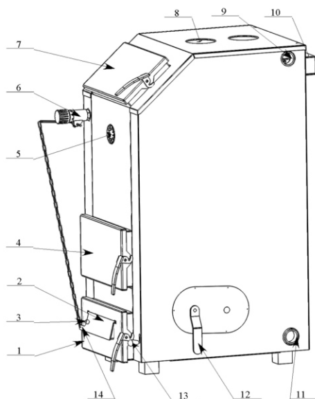
Рис. № 1 Схема устройства котла «Магнум» 15-20 кВт
