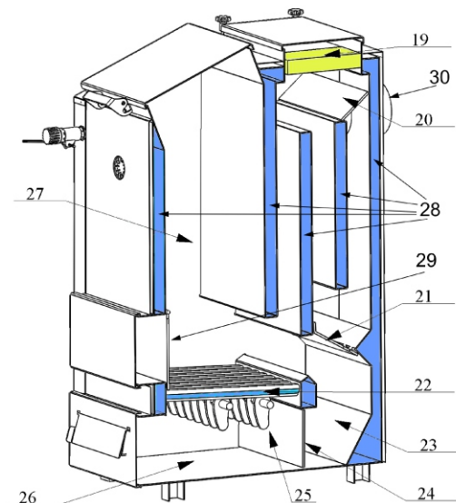
Рис. №5 Схема котла «Магнум» 30 кВт в разрезе
