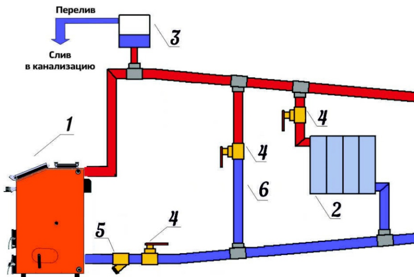
Рис.№7 Подключения котла к открытой системе с естественной циркуляцией теплоносителя:
