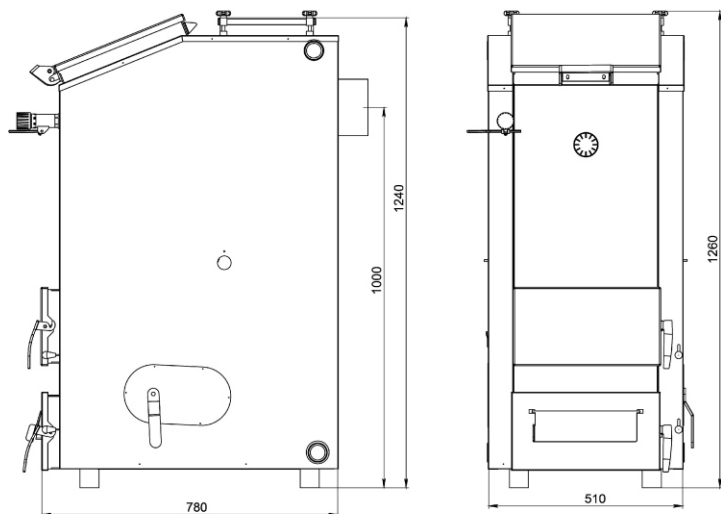
Рис.3 Габаритные размеры котла «Магnum» 30 кВт
