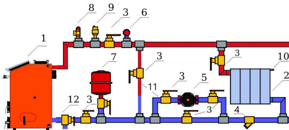
Рис.№10 Подключения котла к 2-х трубной закрытой системе с принудительной циркуляцией теплоносителя:
