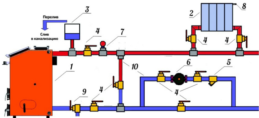
Рис.№9 Подключения котла к однотрубной открытой системе с принудительной циркуляцией теплоносителя:
